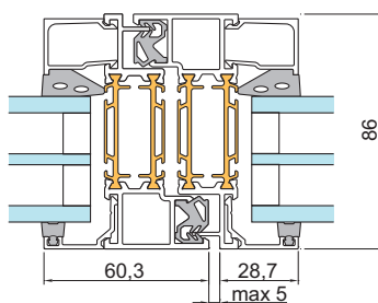
6 - Fast fönster delningsprofil 1086
