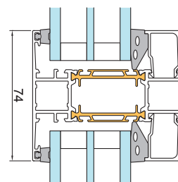
3 - Horisontell spröjs 1086
