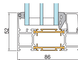
5 - Fast fönster, karm 1086
