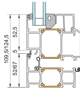
2 - Karm/stor båge Båge till fönsterdörr
