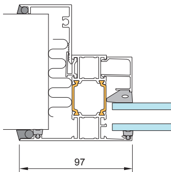
2 - Karm, sida med invändiga foder i lättvägg
