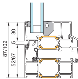
2 - Karm/liten båge
