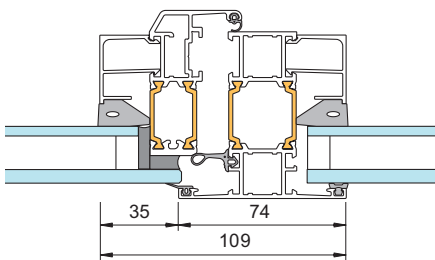
2. Öppningsbart/fast fönster
