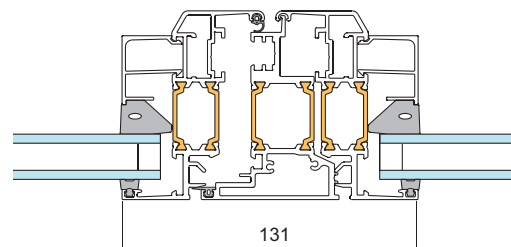
3. Mötesfönster utan mittpost
