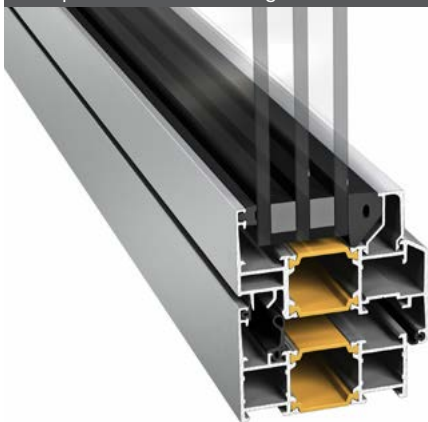
1. Sapa Fönster 1074 inåtgående
