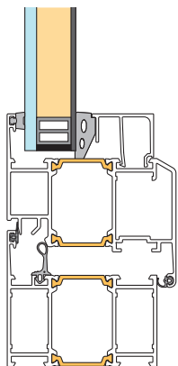
Båge, fyllning med vakumpanel.
