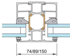
3 - Spröjsprofil
