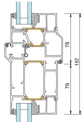
2. Stor båge fast över-/sidoljus
