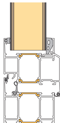
Båge med fyllning
