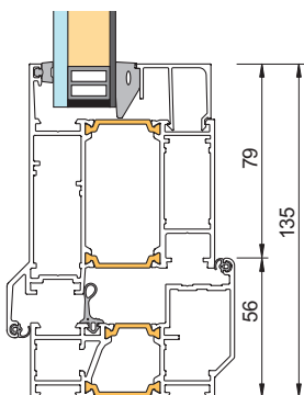
Dörrblad, fyllning med vakumpanel
