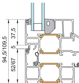
2 - Karm/mellanbåge
