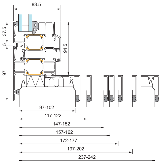
1 - Karm med invändiga foder i lättvägg
