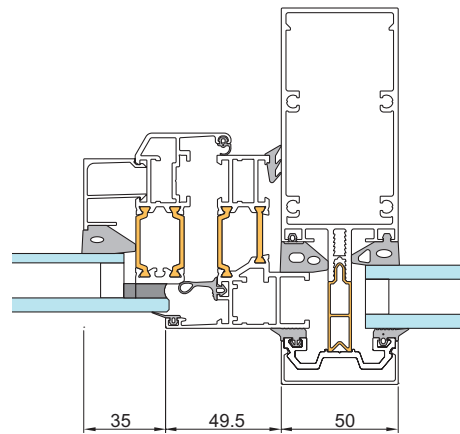
Blockfönster i fasad 4150
