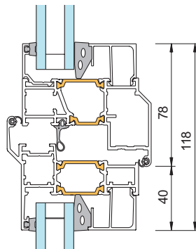
2. Liten båge fast över-/sidoljus (endast motordrift)
