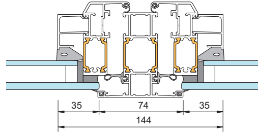
3. Öppningsbart med fast mittpost
