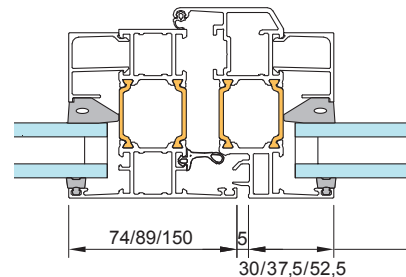
4 - Spröjs med bågprofil
