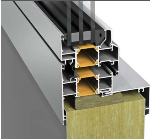
3. Sapa Fönster 1074 inåtgående lättvägg
