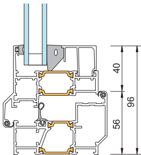
1. Karm med liten båge (endast motordrift)
